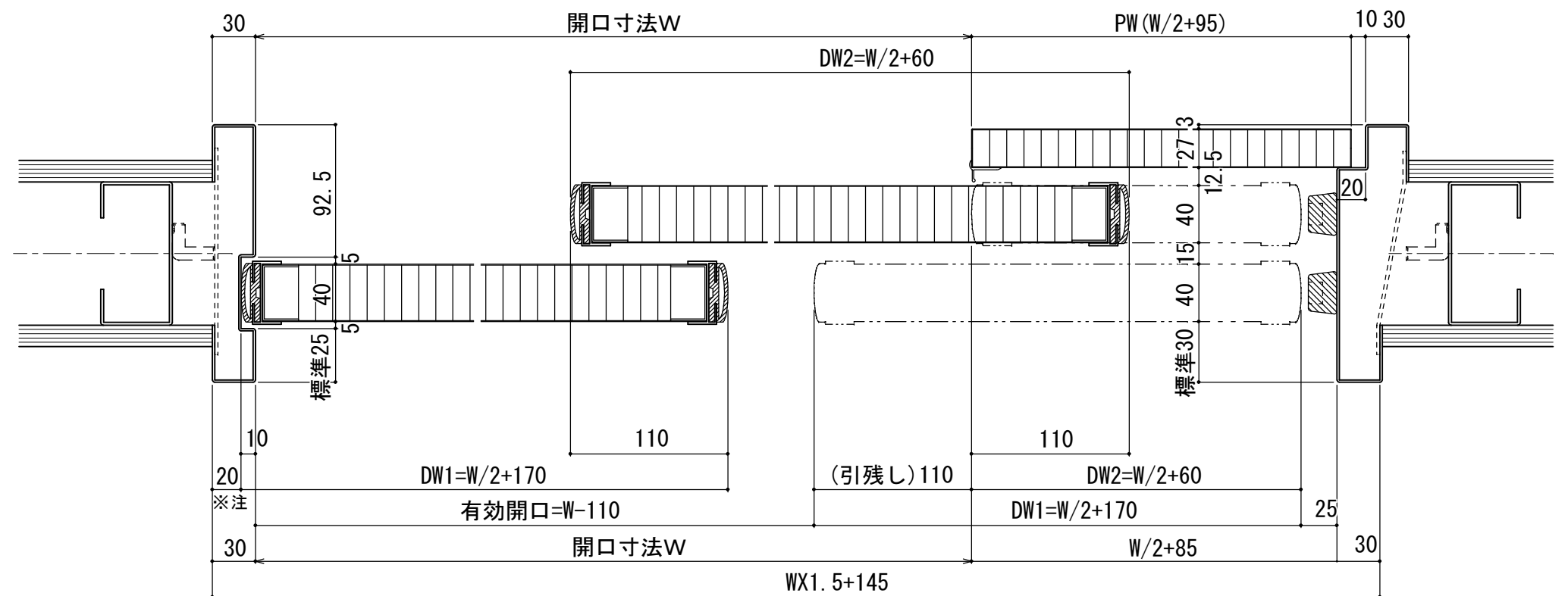
2連式戸袋タイプ右引横断面図
