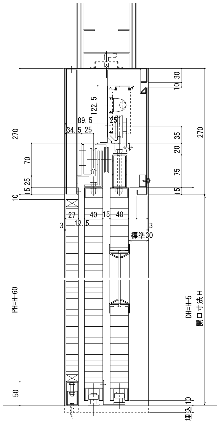
2連式戸袋タイプ縦断面図
